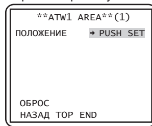
Экран настройки участка
