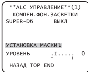
Экран "ALC УПРАВЛЕНИ"
