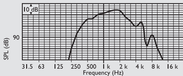
Частотная характеристика
