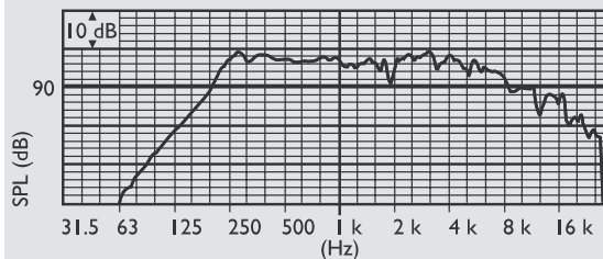
Частотная характеристика
